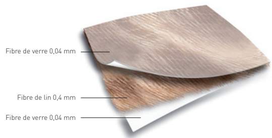
> Membrane sandwich en fibre de lin Constitution d'un cône pour haut-parleur médium
